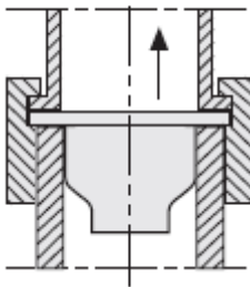
Installation av backventil i inloppsröret för kallvatten beroende på version.
